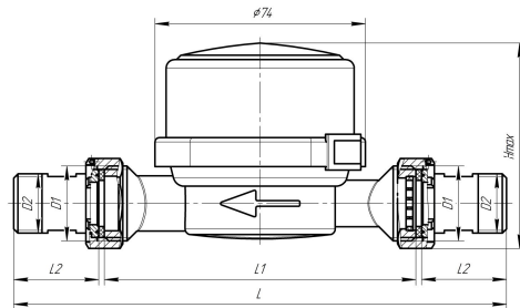
Рисунок 1. Габаритные и присоединительные размеры счетчиков воды СХВЭ, СГВЭ
